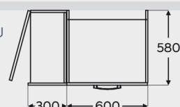
Columna final con marco ALU SWAR30x58/71
